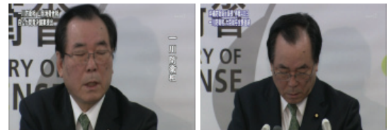
図 11 誤検出例
