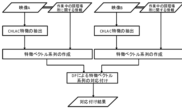
図 3 処理の流れ
