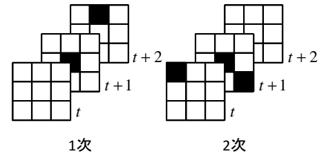
図 4 CHLAC 特徴の変位パターンの例
